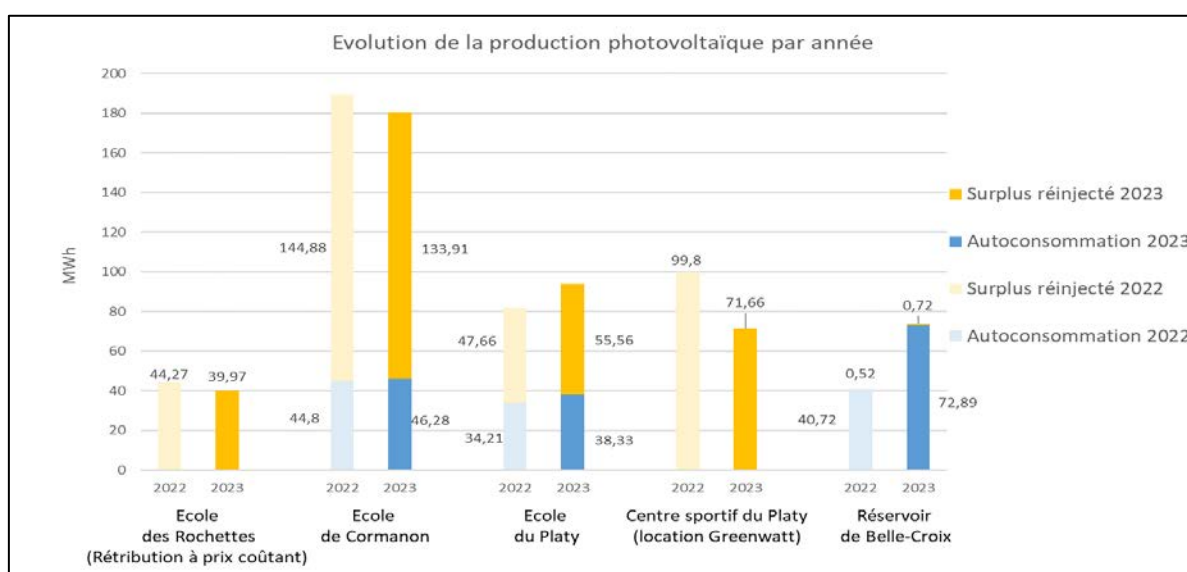
Evolution de la production photovoltaïque (2022-2023)
